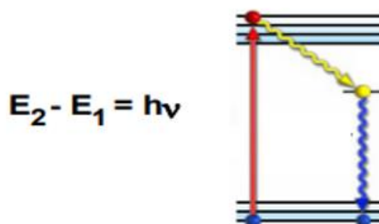
Figura 9. Diagrama de niveles de energía en una molécula
