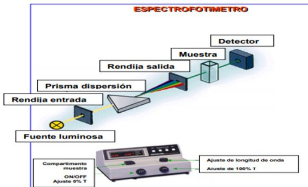
Figura 11: Componentes espectrofotómetro.
