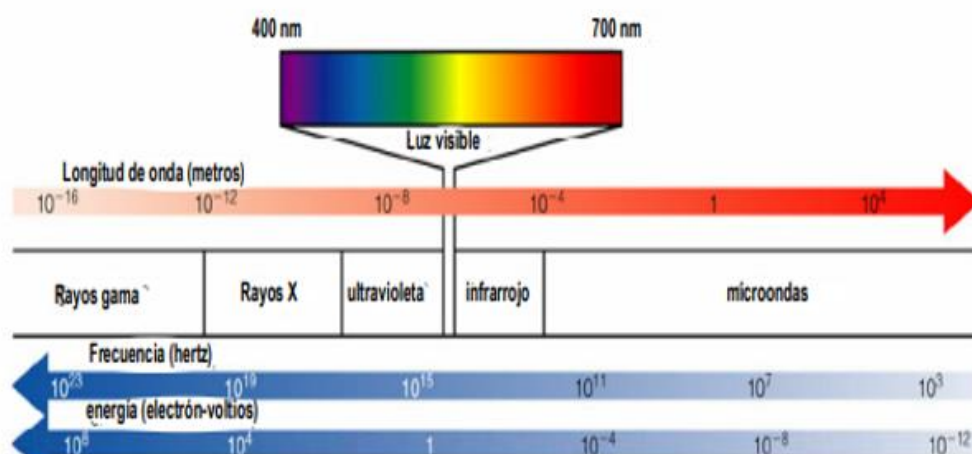
Figura 10. Espectro electromagnético
